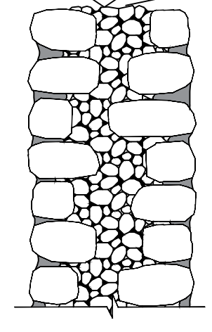
פרט יישום קופינג קנ"מ 1:20
