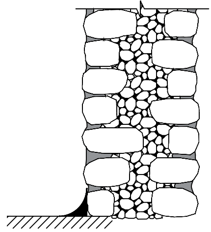
פרט יישום רולקה קנ"מ 1:20
