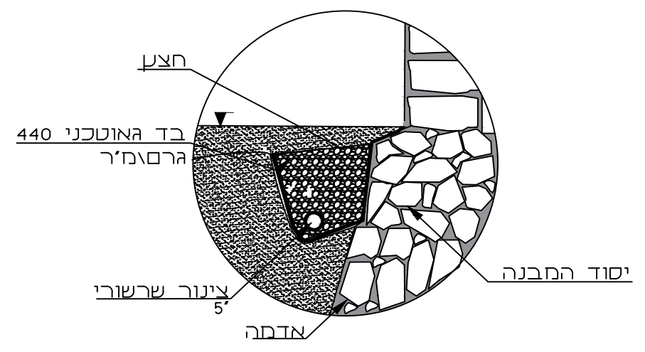
פרט ניקוז היקפי
