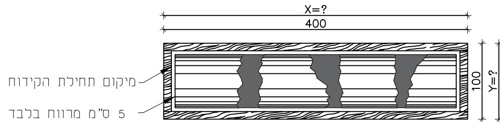
תכנית ארגז לצורך שמירת הגליל מידות הארגז מתאים למידות הגליל לאחר הזרקת גראוטינג
