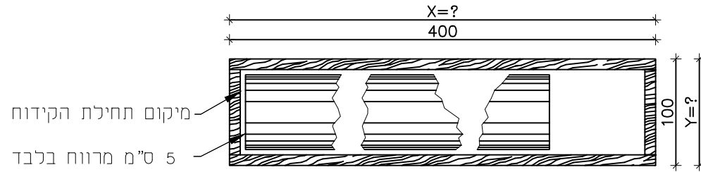
תכנית ארגז לצורך שמירת הגליל מידות הארגז מתאים למידות הגליל לפני הזרקת גראוטינג
