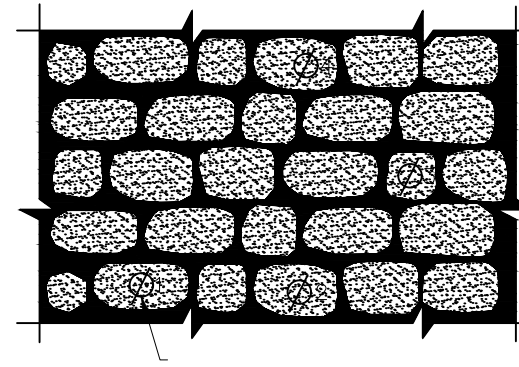
מיקום הוצאת קורים/גלילים <math>\phi 2''</math> לבדיקה אורך הגליל כאורך הקיר
