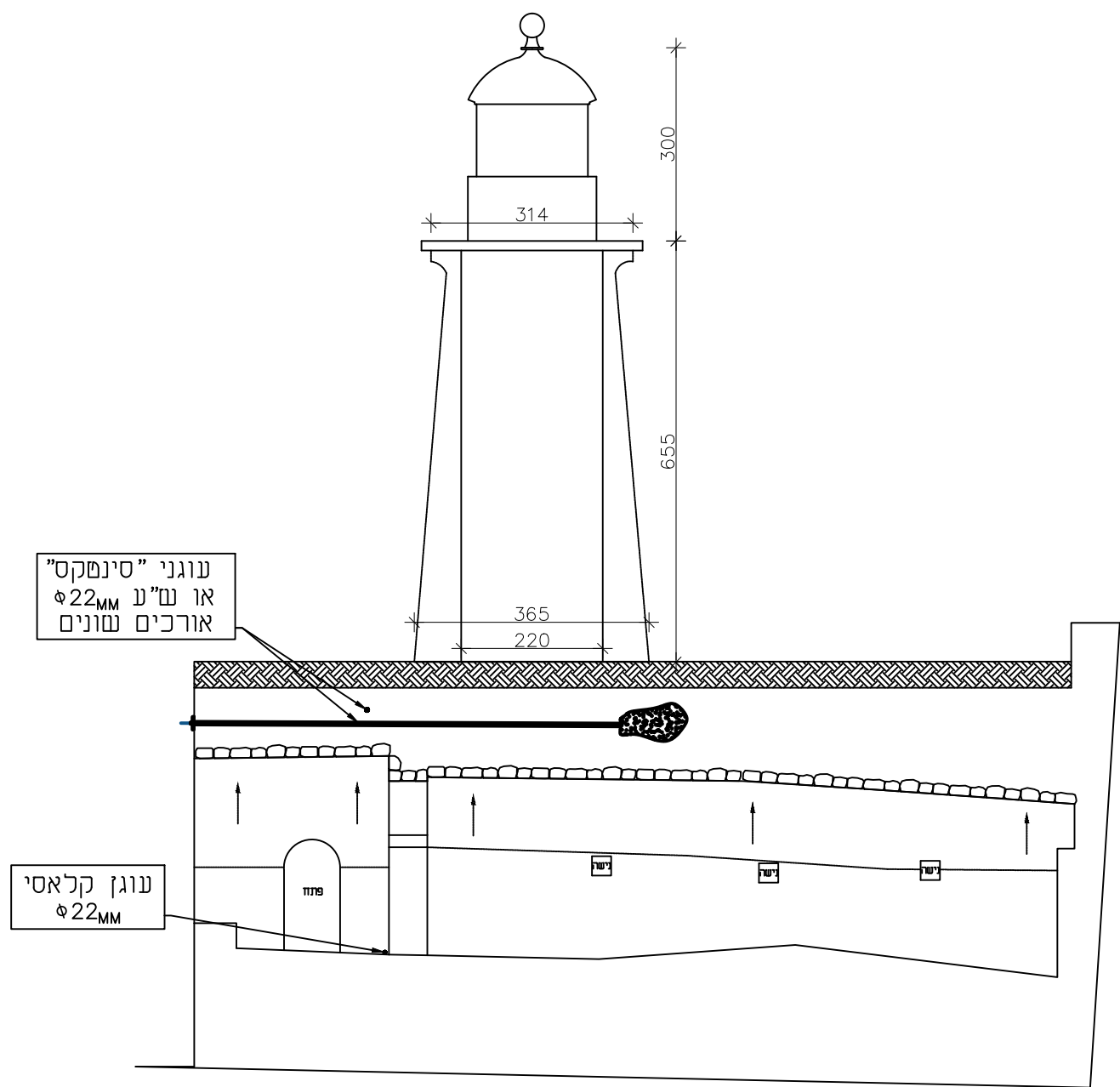
חתך 6-6 מיקום עוגנים קנ"מ: 1:100
